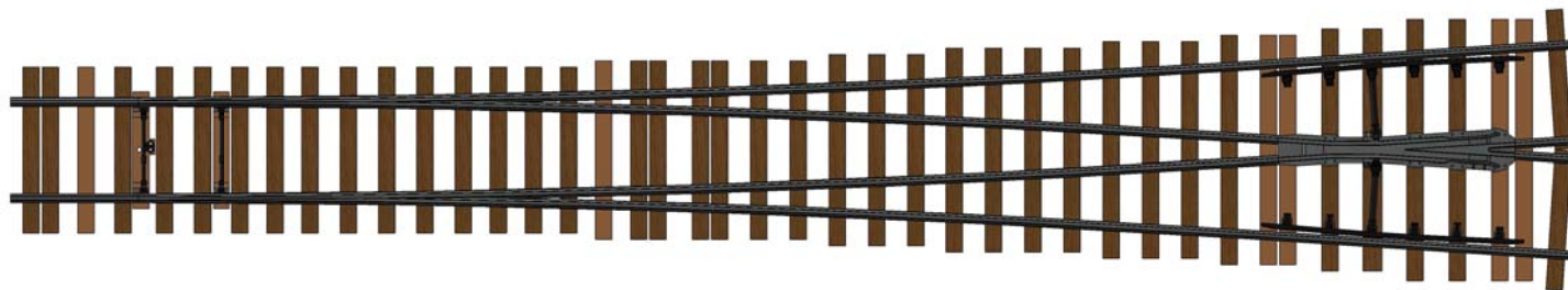
Branchement symétrique, modèle partiellement monté échelle 2/3
