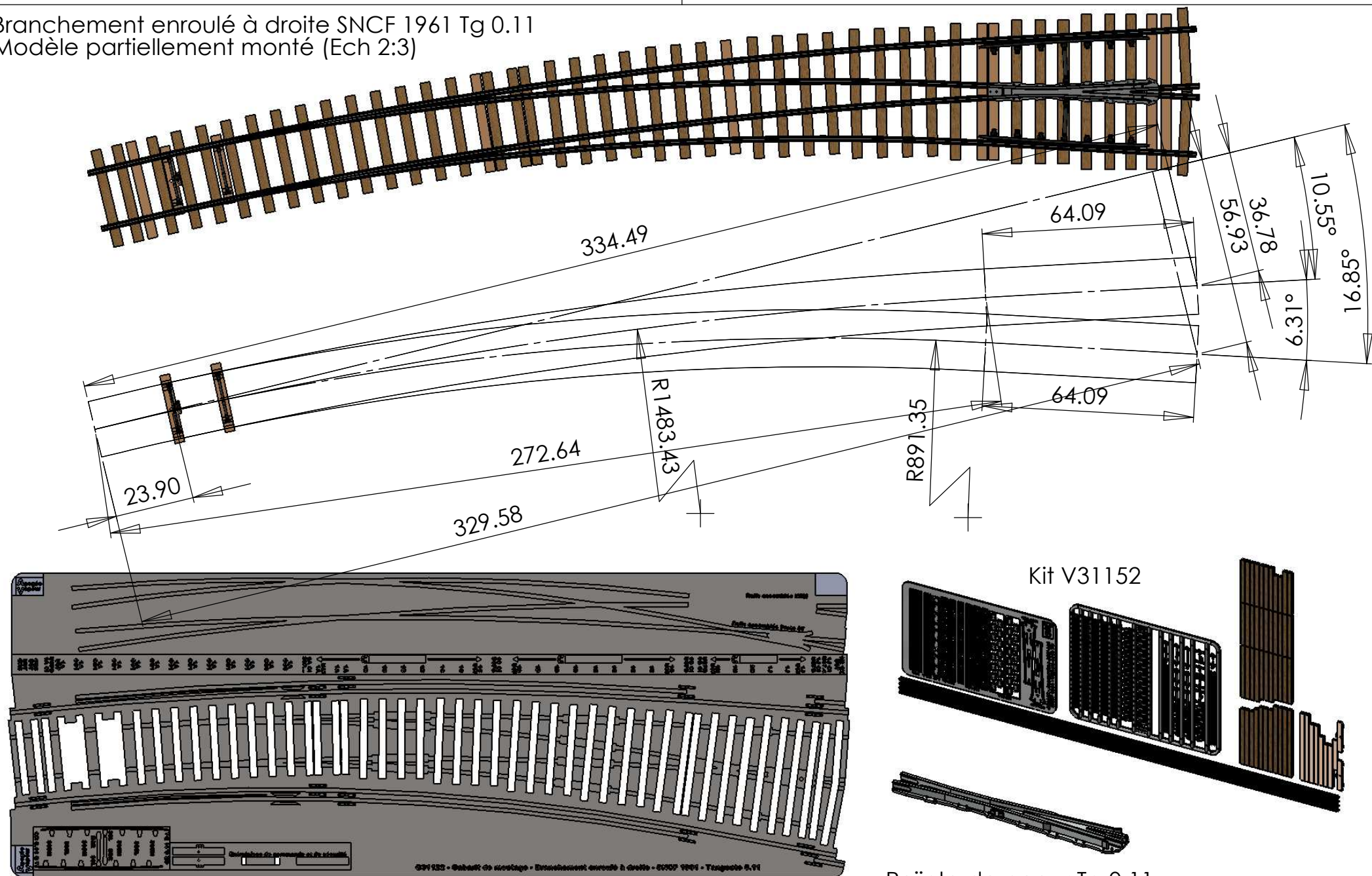
Gabarit G31122 (Ech 1:2)
