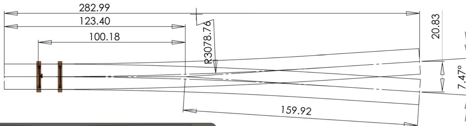
Branchement symétrique, modèle partiellement monté échelle 2/3
