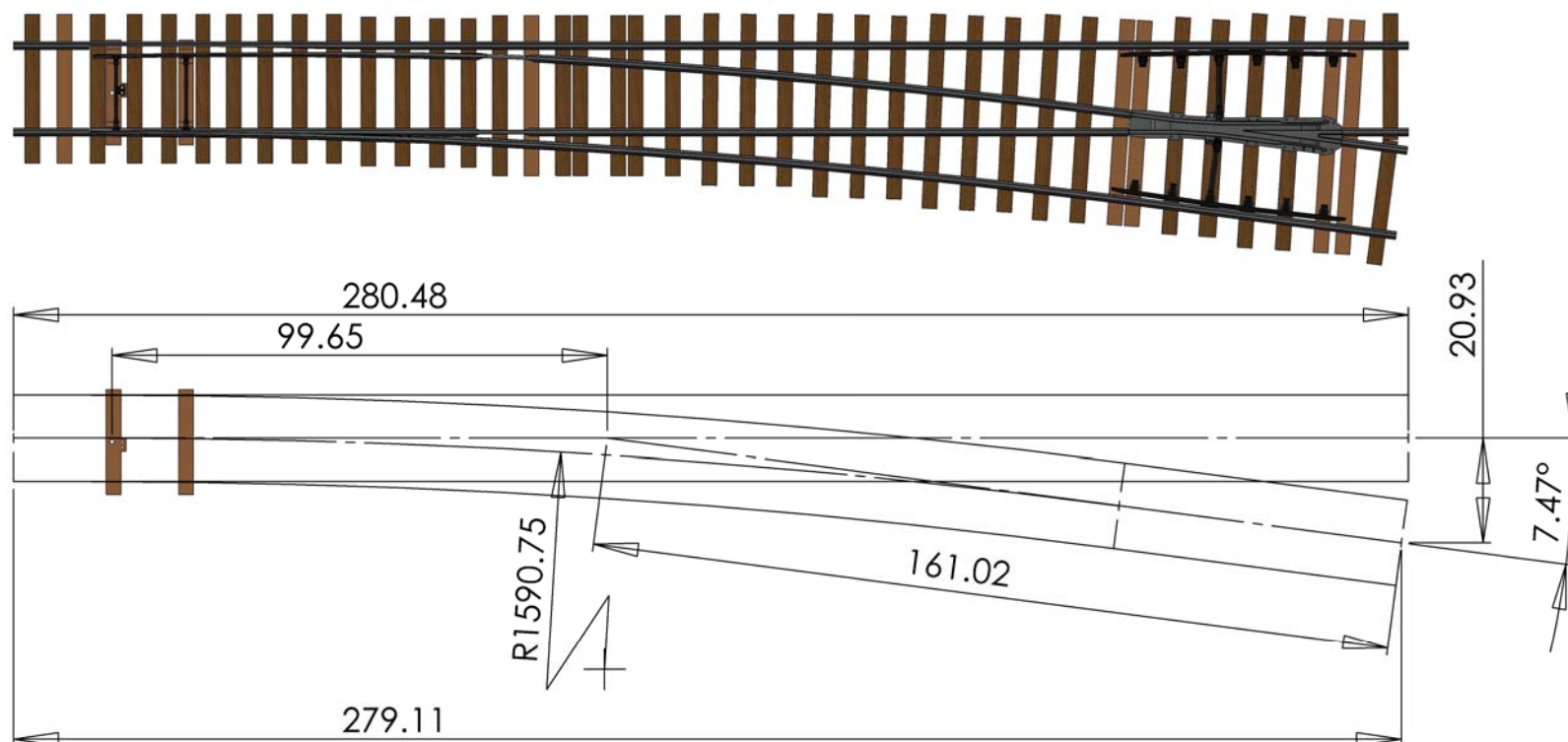
Kit V31150
