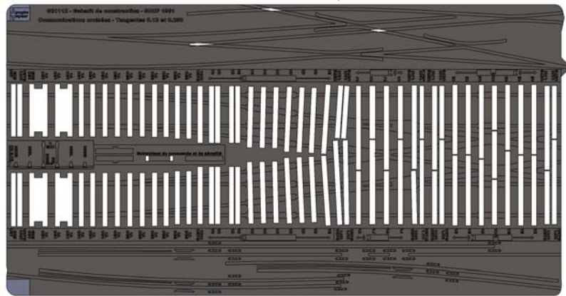
Gabarit G31112
